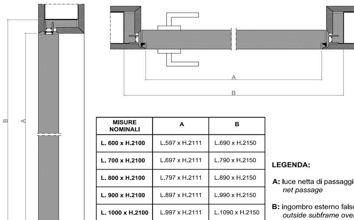
SEZIONE ORIZZONTALE horizontal section
