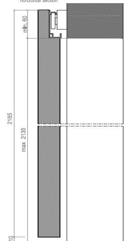
SEZIONE ORIZZONTALE horizontal section
