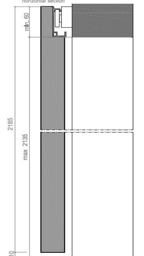
SEZIONE ORIZZONTALE horizontal section
