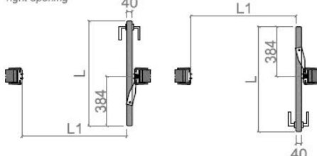
APERTURA DESTRA right opening
