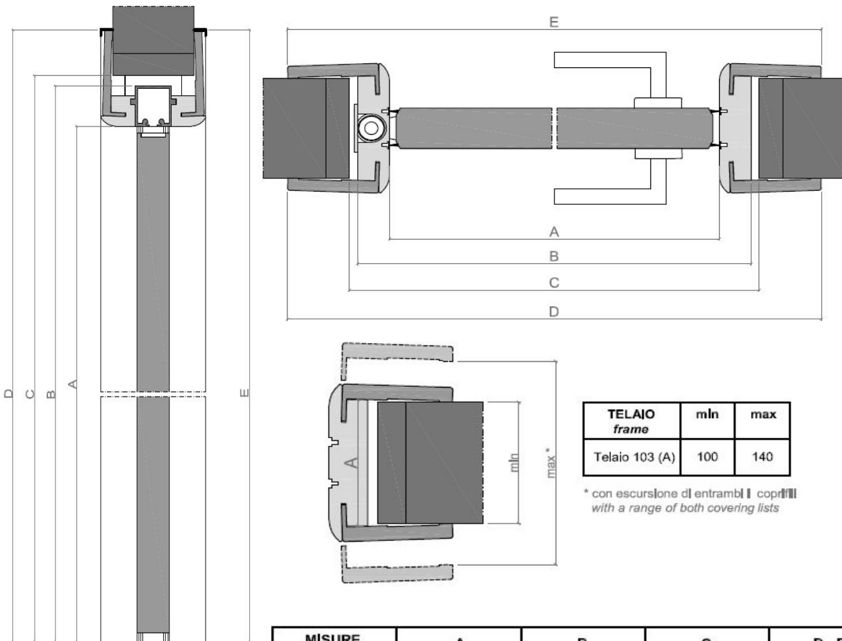
SEZIONE VERTICALE vertical section
