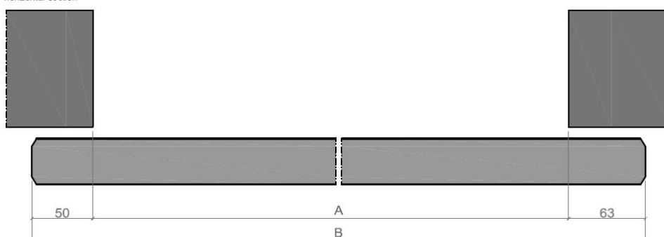
SEZIONE ORIZZONTALE horizontal section
